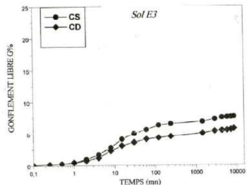
Figure 5 : Evolution du potentiel de gonflement en fonction du temps et du mode de compactage
