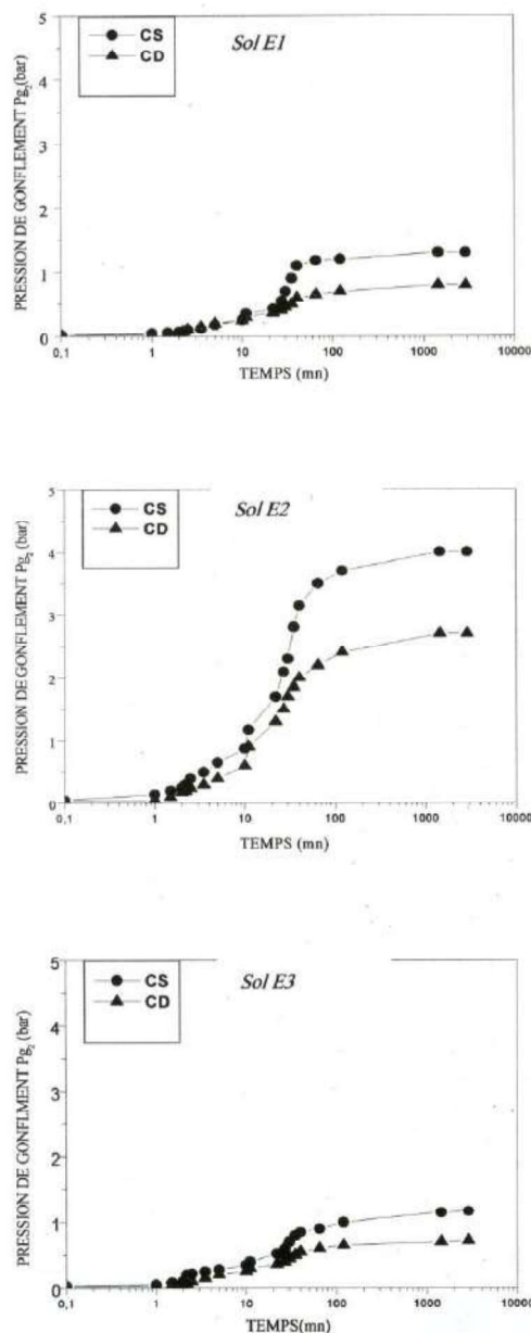
Figure 6 : Evolution de la pression de gonflement en fonction du temps et du mode de compactage
