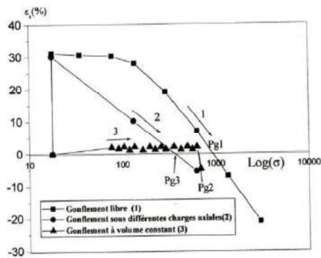
Figure 4 : Différentes procédures d'essais de pression de gonflement (Sridharan et al. 1986)
