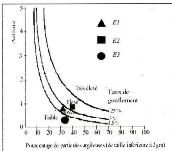
Figure 2 : Abaque d'évaluation du potentiel de gonflement (Seed, 1962)
