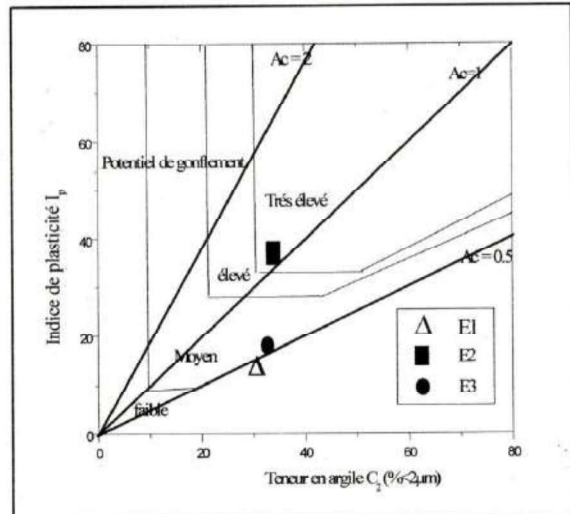
Figure 3 : Classification des potentiels de gonflement (Williams & Donaldson 1980).
