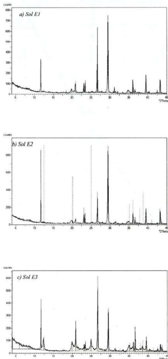
Figure.1 : Analyse minéralogique des sols
